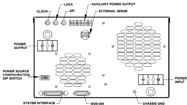
2750L / 4500L / 6000L REAR PANEL
