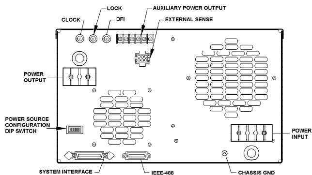
2750L / 4500L / 6000L REAR PANEL
