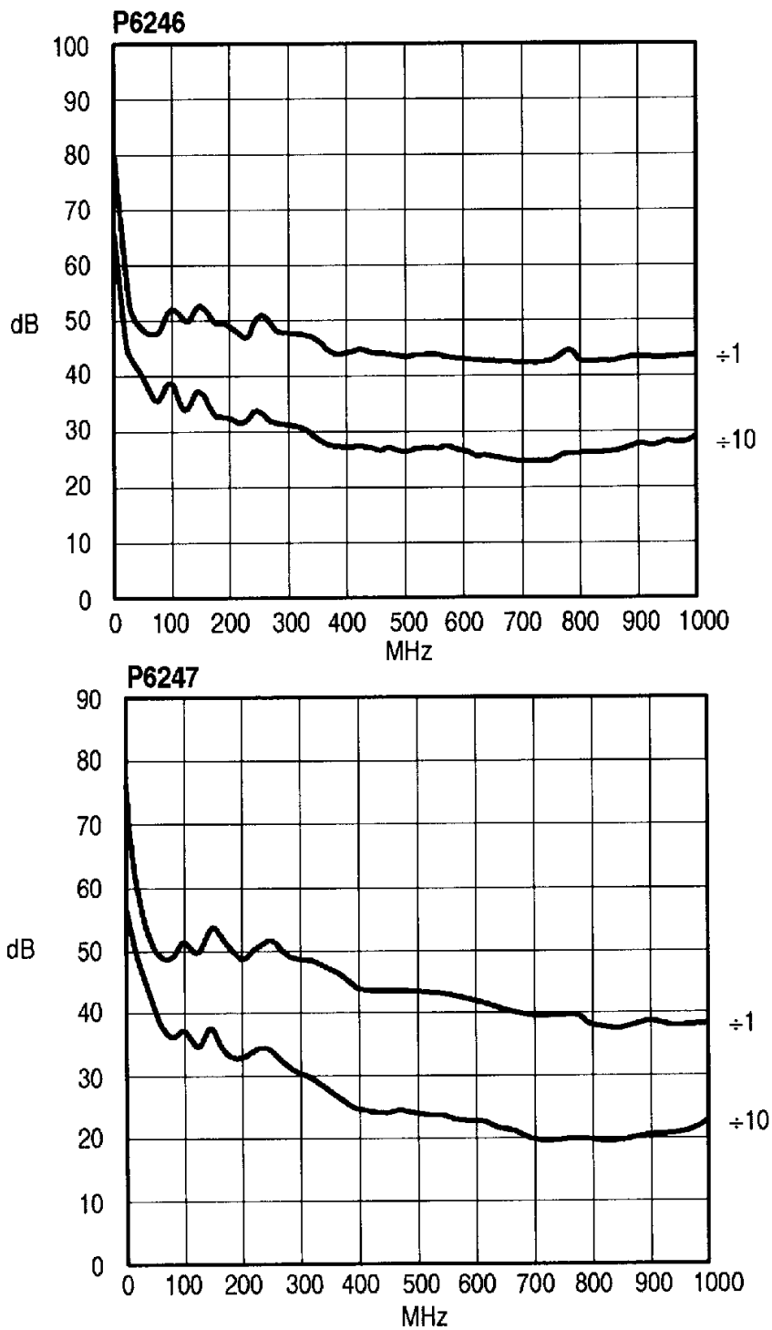
그림 8. 일반 동상 제거비(감쇠율 \div 1 과 \div 10 )
