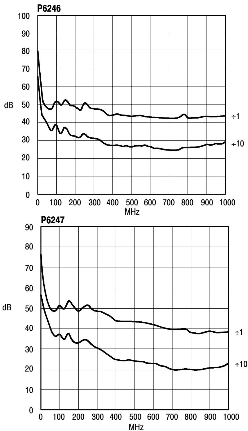
Figure 8 : Taux de réjection en mode commun type (atténuation \div 1 et \div 10 )
