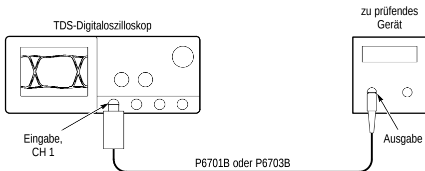
Abbildung 3: Anordnungen mit TekProbe II-Schnittstelle
