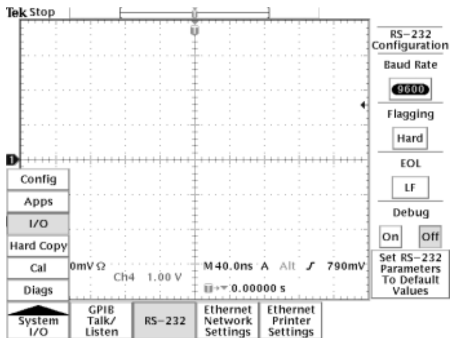
Figure 1–19: RS-232 parameter settings
