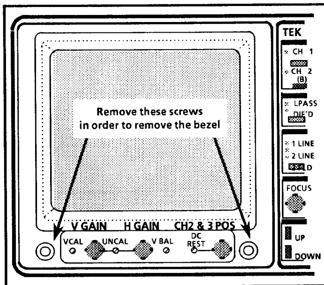
Fig. 6-4. Bezel Securing Screws
